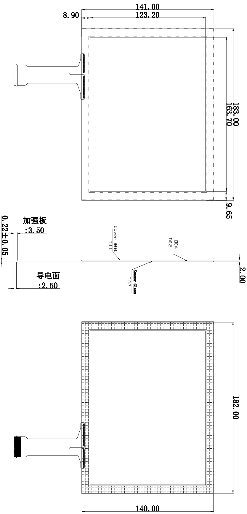
正视图
