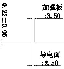
侧视图
