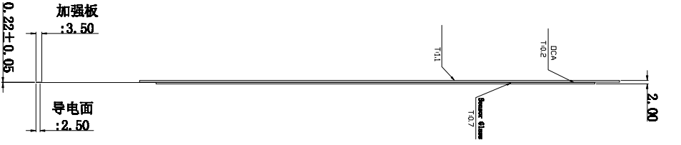
侧视图
