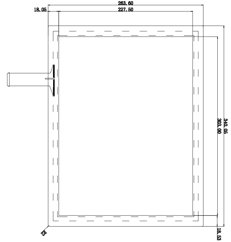
正视图
