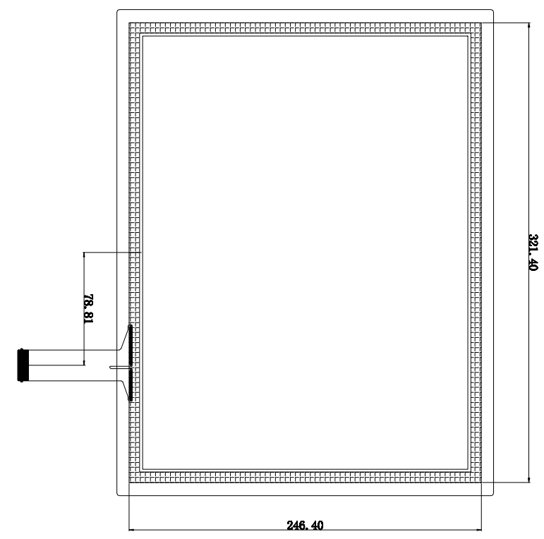
背视图
