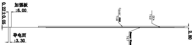
侧视图
