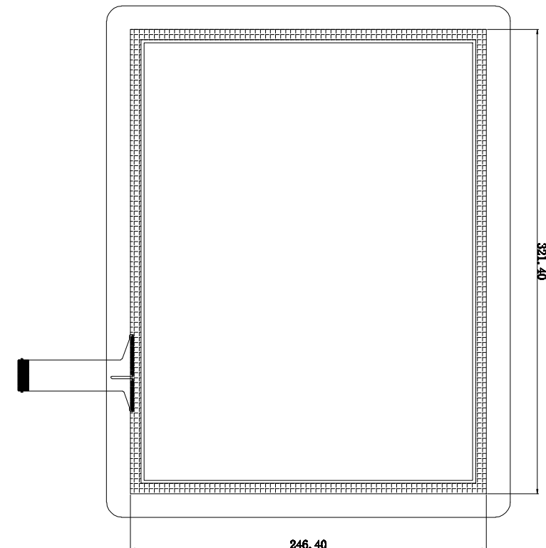
背视图
