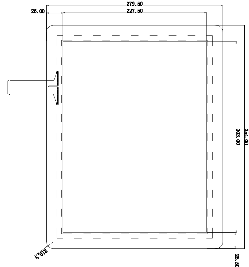
正视图
