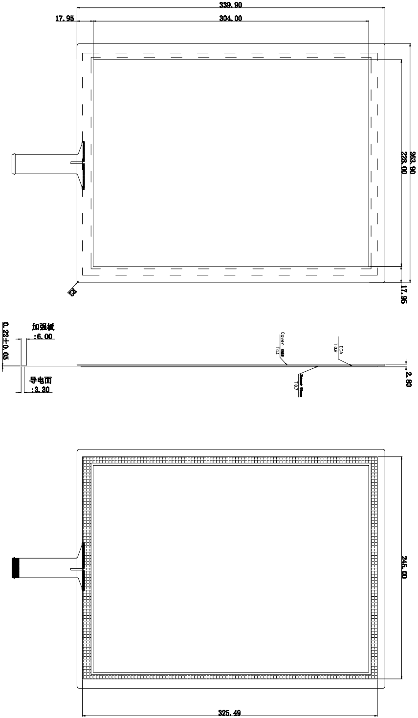
正视图
