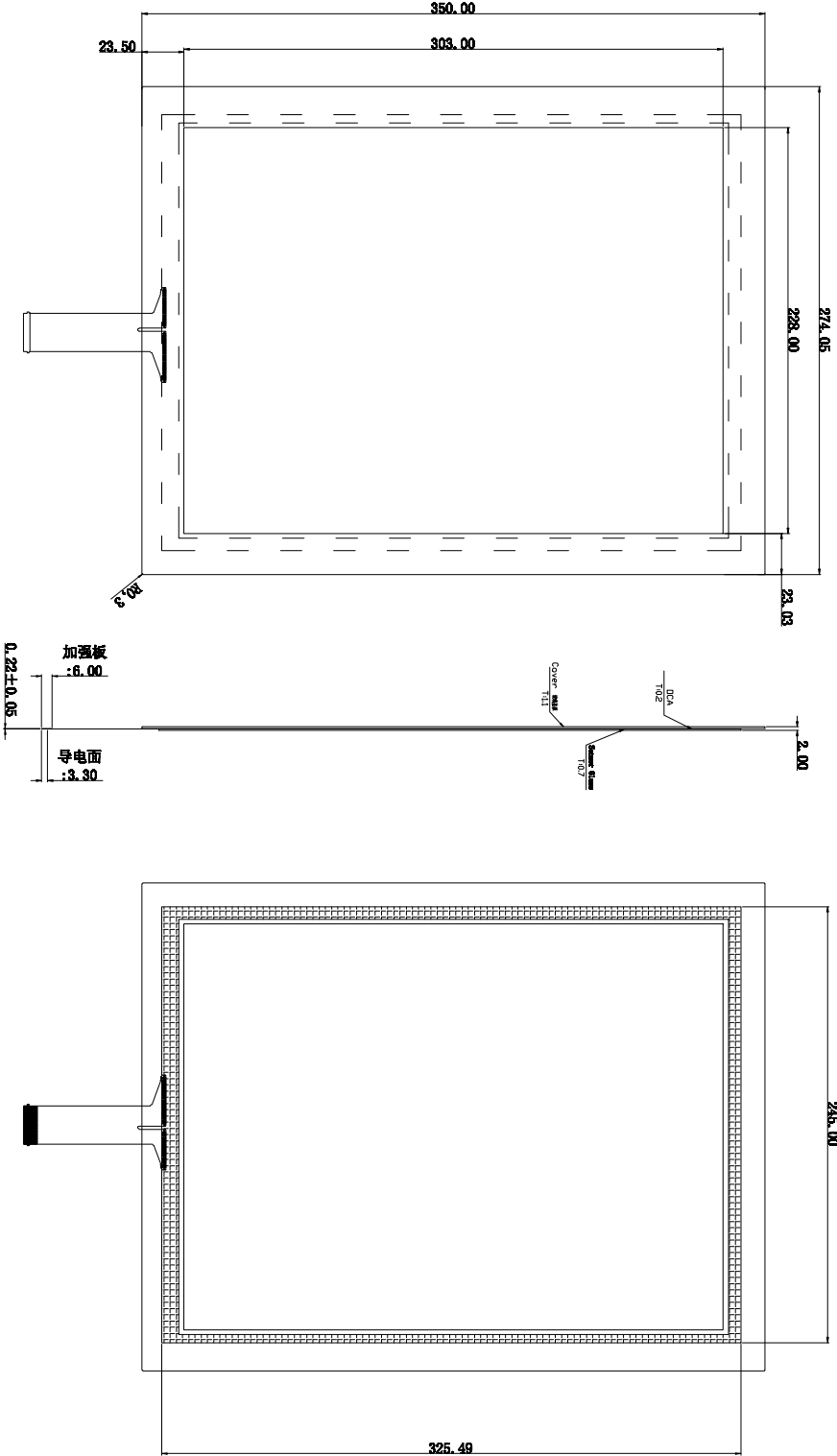
正视图
