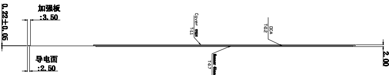
侧视图
