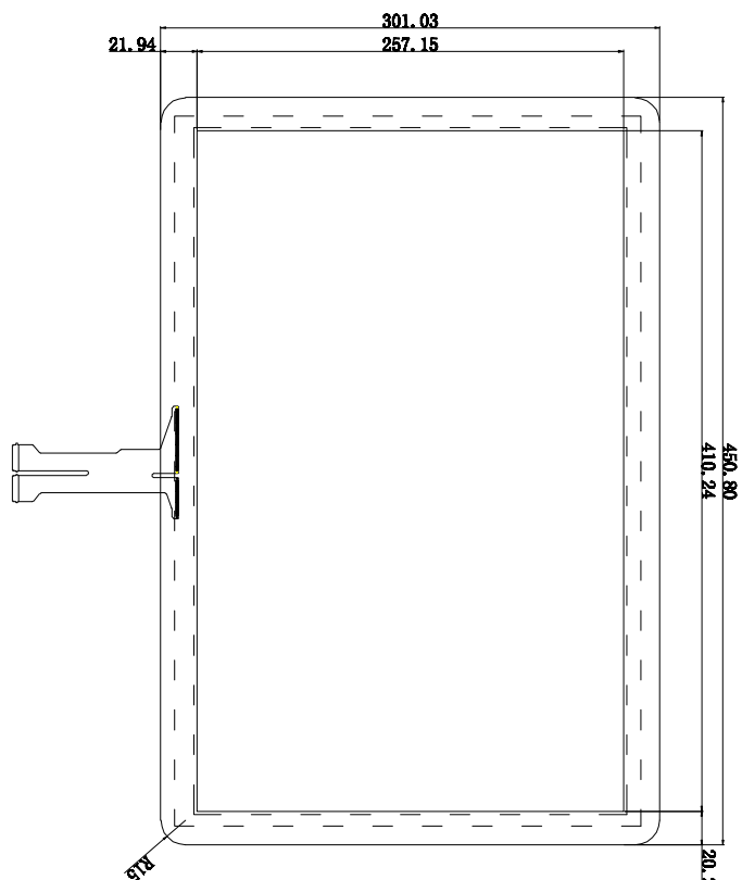
正视图
