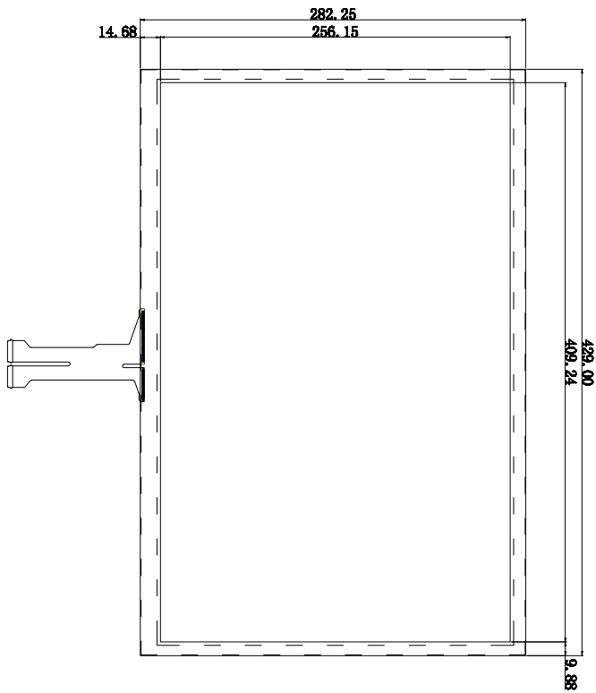
正视图
