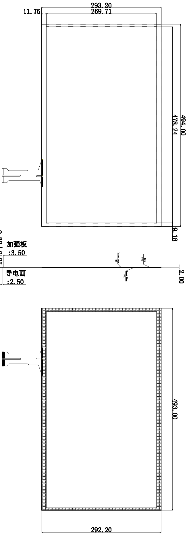
正视图
