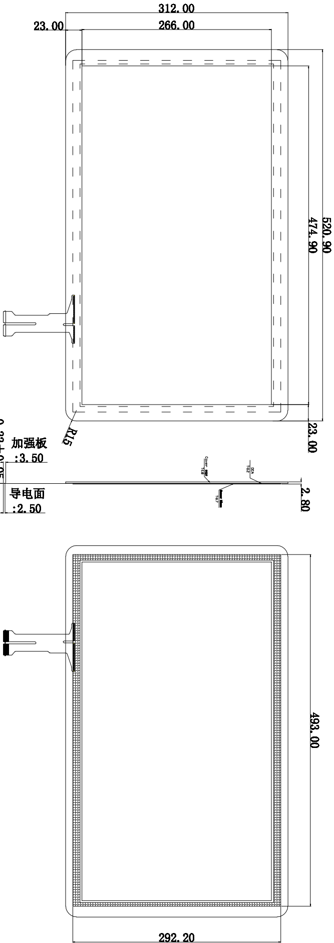
正视图
