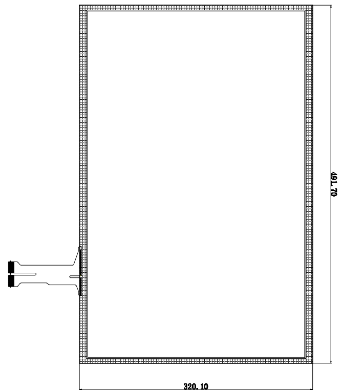
背视图
